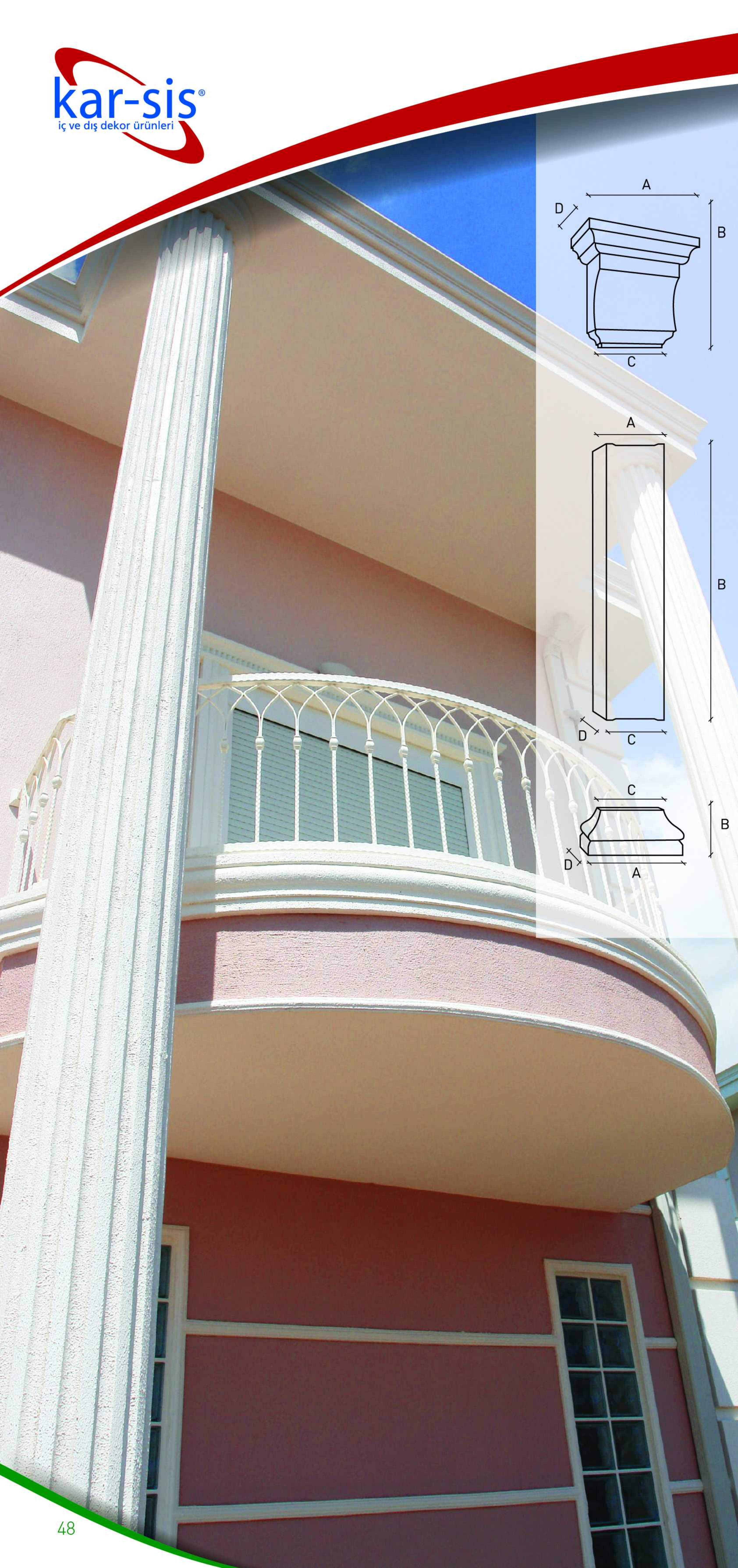
DIŞ 151 A: 20cm B: 200cm C: 20cm D: 3cm
