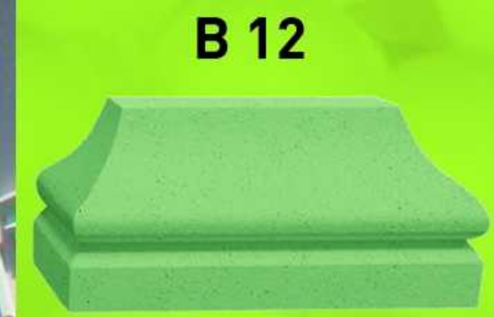
B 12 A: 37cm B: 15cm C: 23cm D: 12cm
