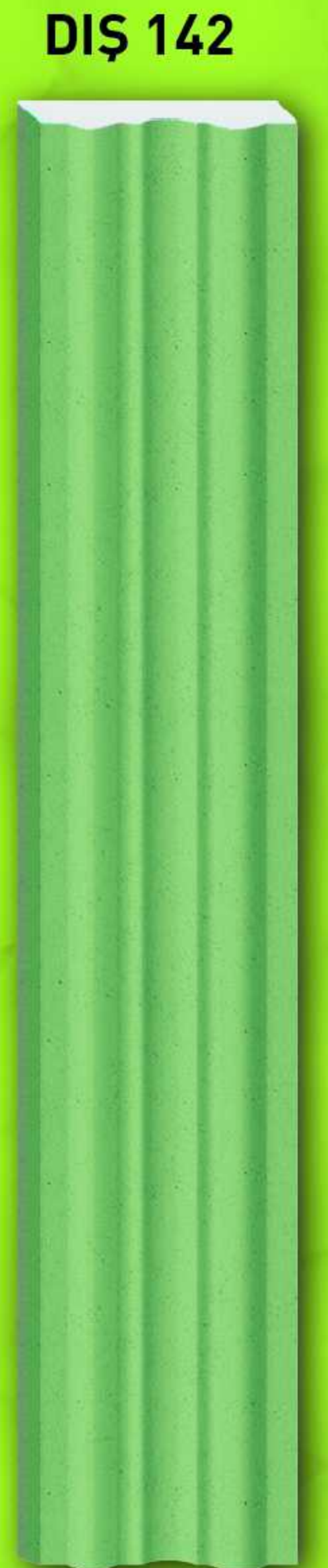
DIŞ 142 A: 20cm B: 200cm C: 20cm D: 4cm
